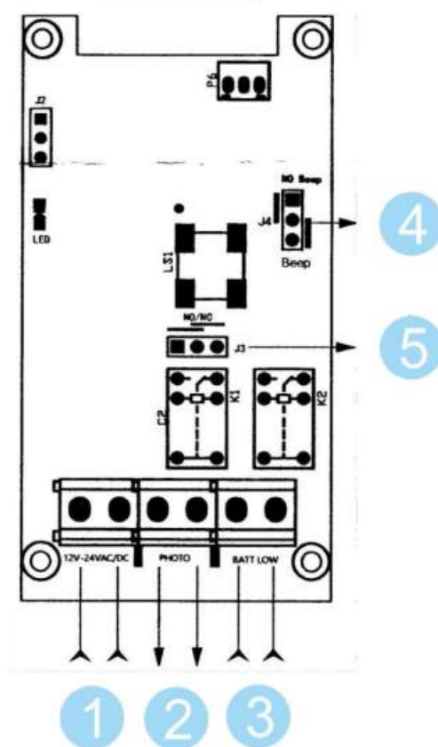
Рисунок 35. Устройство платы приемника
