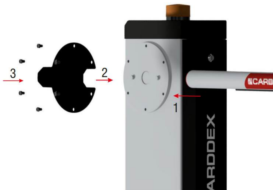
Рисунок 26. Установка стрелы на шлагбаум
