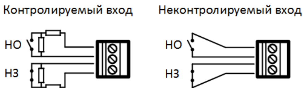
Типы подключения входов контроллера ST-NC441R2
