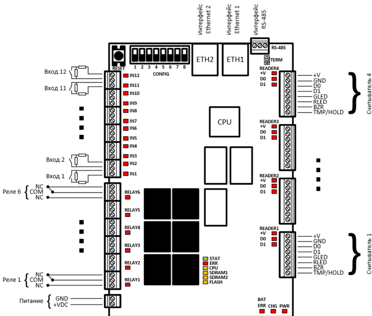
Назначение контактов контроллера ST-NC441R2
