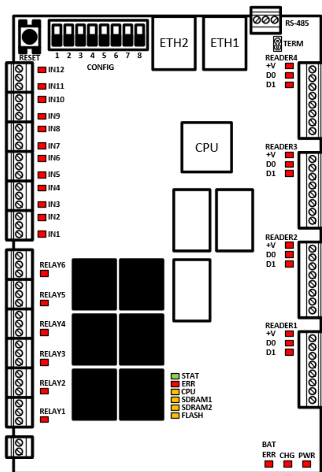
Индикаторы контроллера ST-NC441R2
