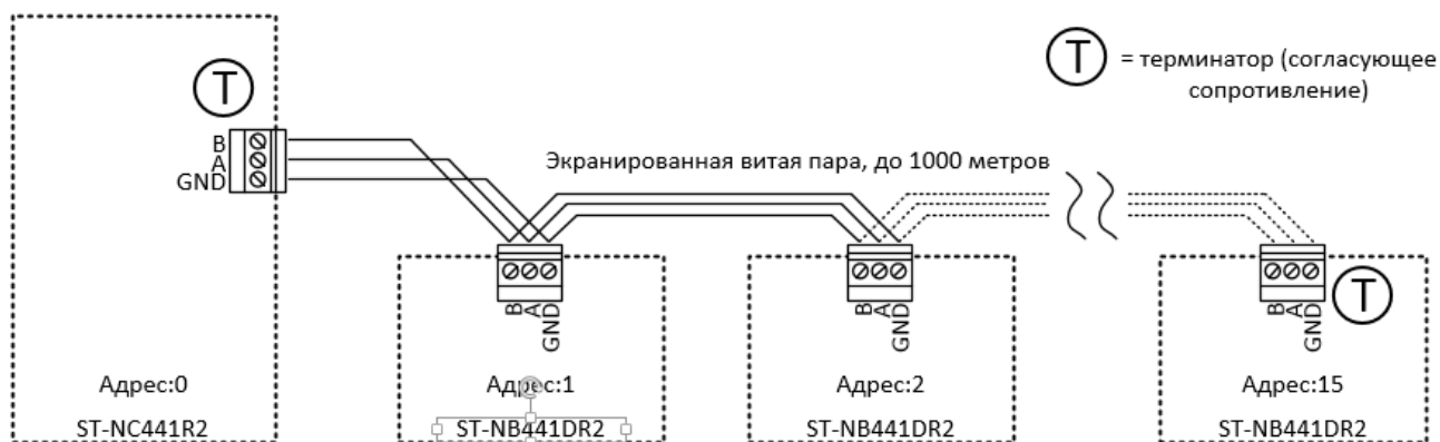
Схема подключения шины RS-485
