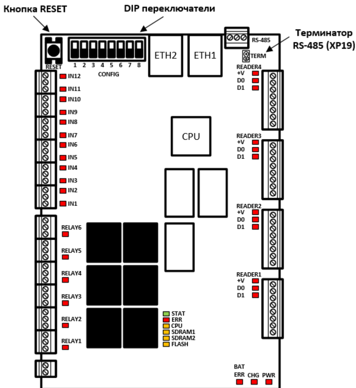
Расположение DIP переключателей на контроллере ST-NC441R2
